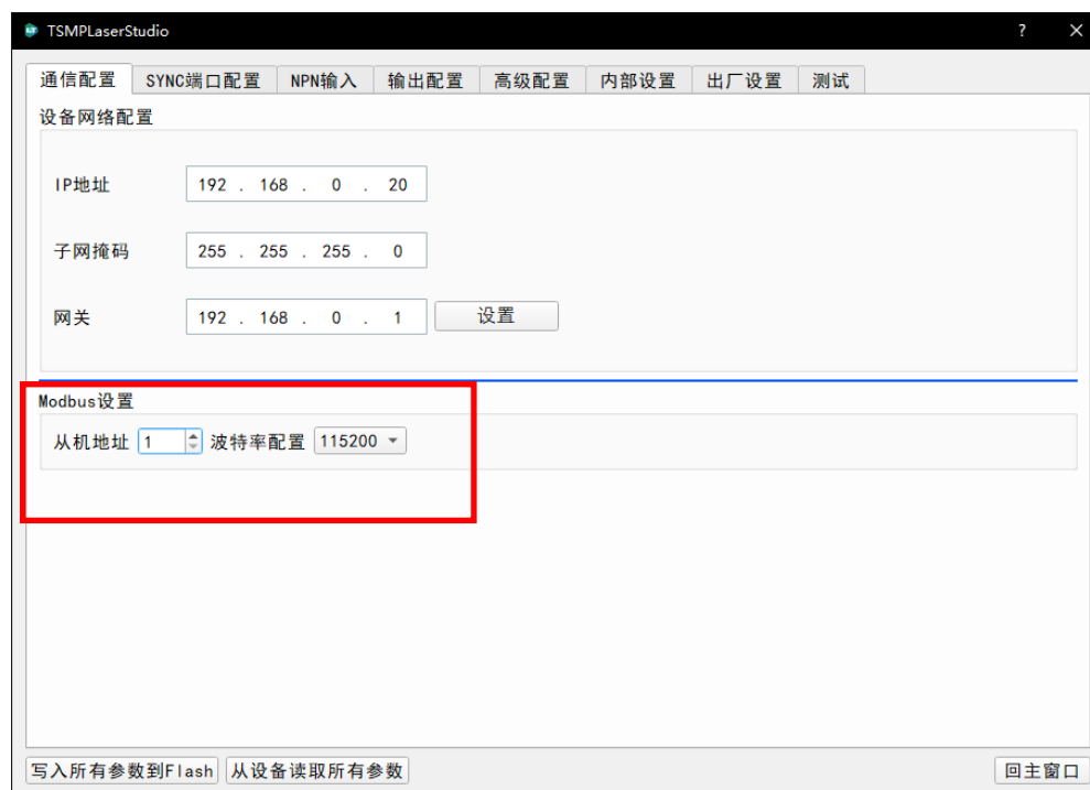
图 6-1 Modbus 通信参数配置
